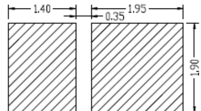
建议焊盘
